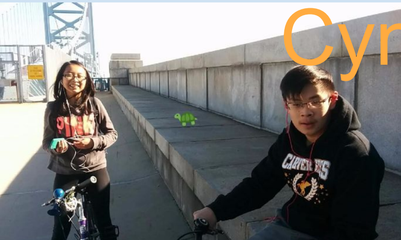
Interpreter
